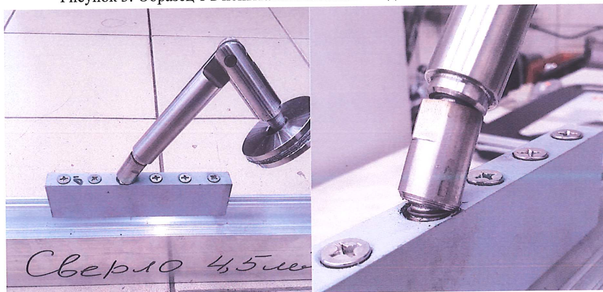
Рисунок 4. Характер разрушения
