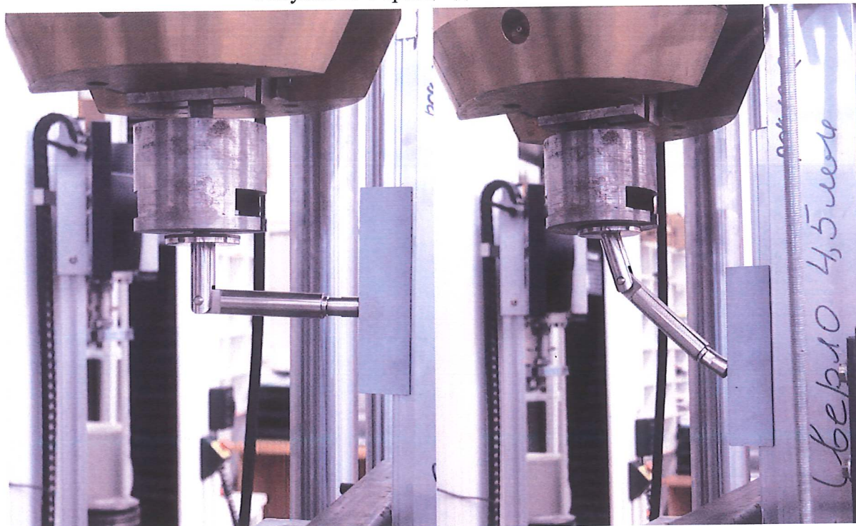
Рисунок 3. Образец 1 в испытательной машине до и после испытания
