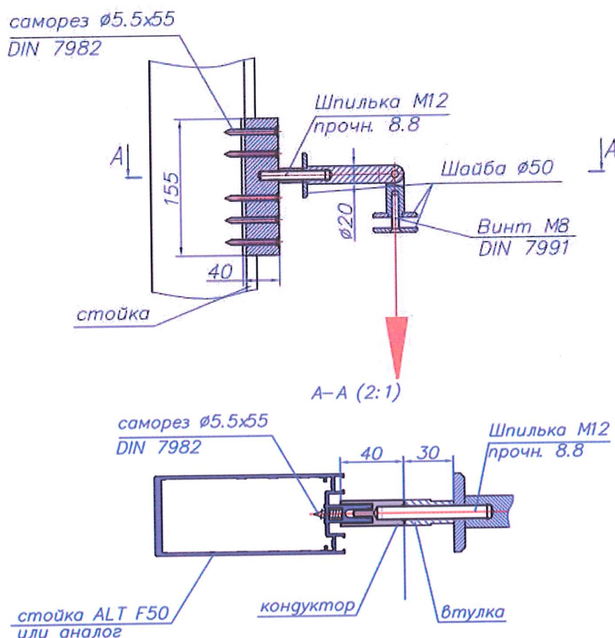
Рисунок 1. Схема испытания на изгиб кондуктора для стоечно-ригельных систем (серия РСК 10)
