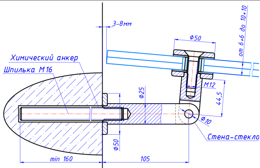
Крепление стена-стекло, РДК-14
