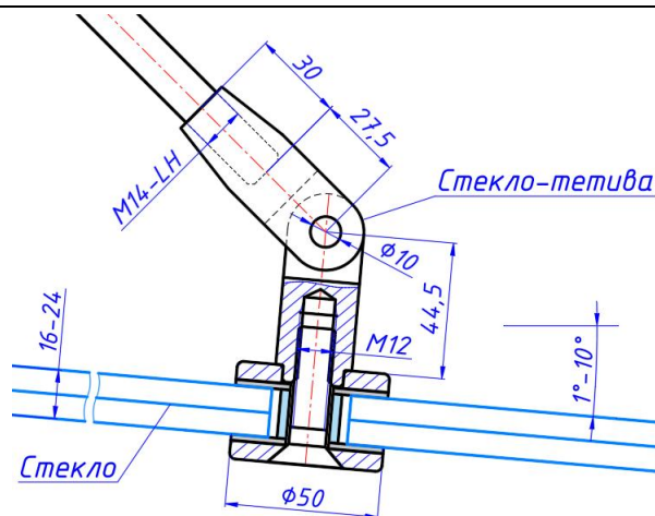
Крепление стекло-тетива, РДК-14
