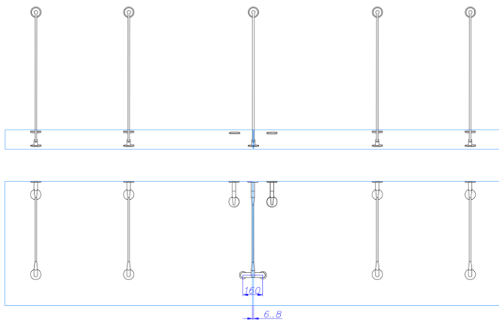
Тип 4 – 2 стекла, 4 комплекта РДК-14 и 1 комплект РДКД-14 (с одним спайдером)
