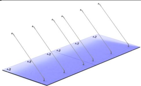
Тип 4 – 2 стекла, 4 комплекта РДК-14 и 1 комплект РДКД-14 (с одним спайдером)
