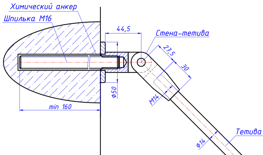
Крепление стена-тетива, РДК-14
