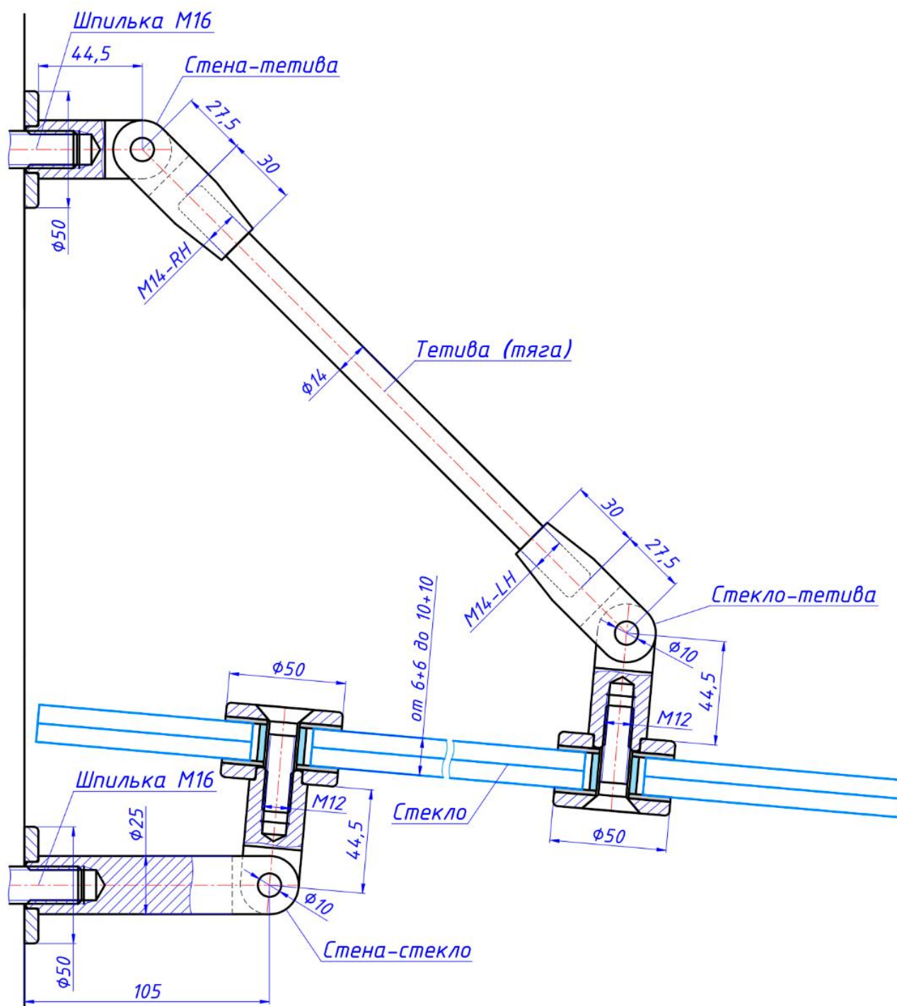
Фурнитура серии РДК-14
