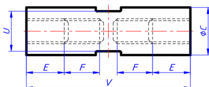
Муфта натяжная
