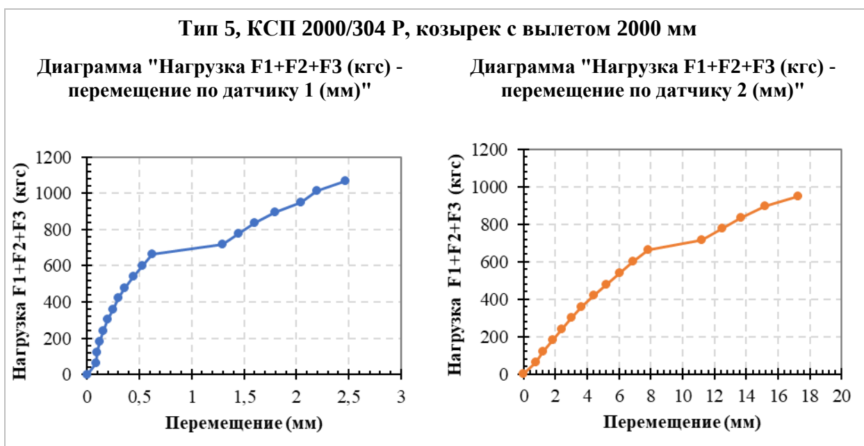
Рисунок 4. Диаграммы "Нагрузка (кгс) – перемещение (мм)" для образца Тип 5
